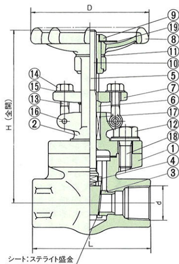
ソケットウエルド形 (SF-SRW)
