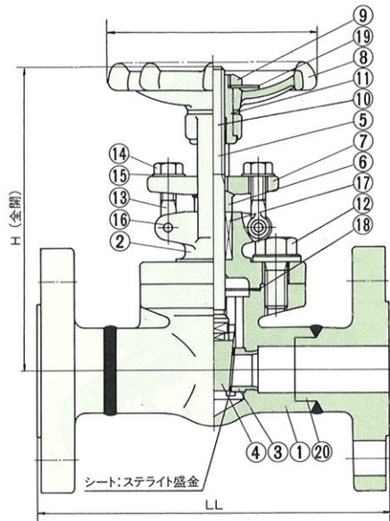
フランジ形 (SF-SRF)
