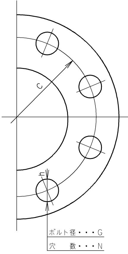
寸法表 単位: mm
