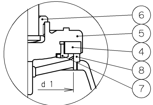
図 1 呼び径6のディスク部の構造
