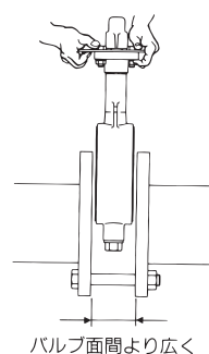
バルブ面より広く
