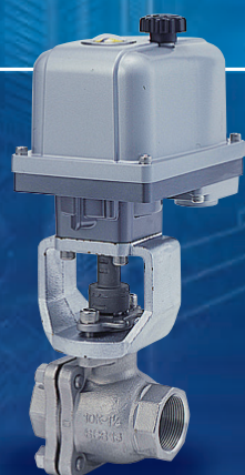
MX型アクチュエータ付 フルボアボールバルブ
