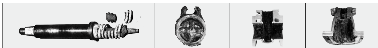
黄銅製ステム（C3771 BE,BD）の脱亜鉛腐食
