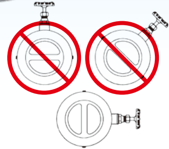
水平配管時の正しい取付姿勢
