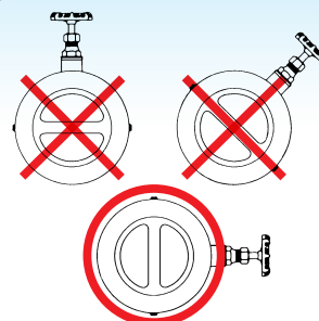
水平配管時の正しい取付姿勢
