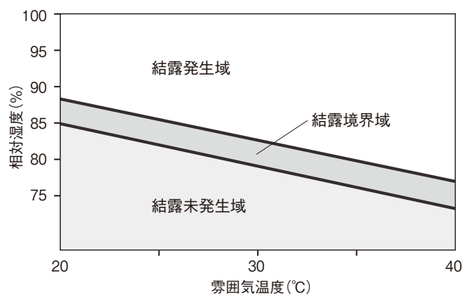
10L2-N-U-EL 600 A 結露境界予測図
