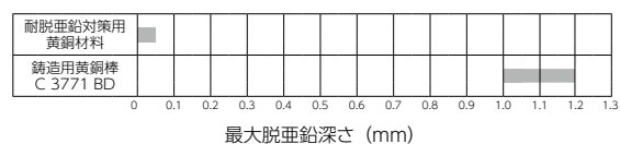
ISO 6509 による脱亜鉛腐食試験結果
